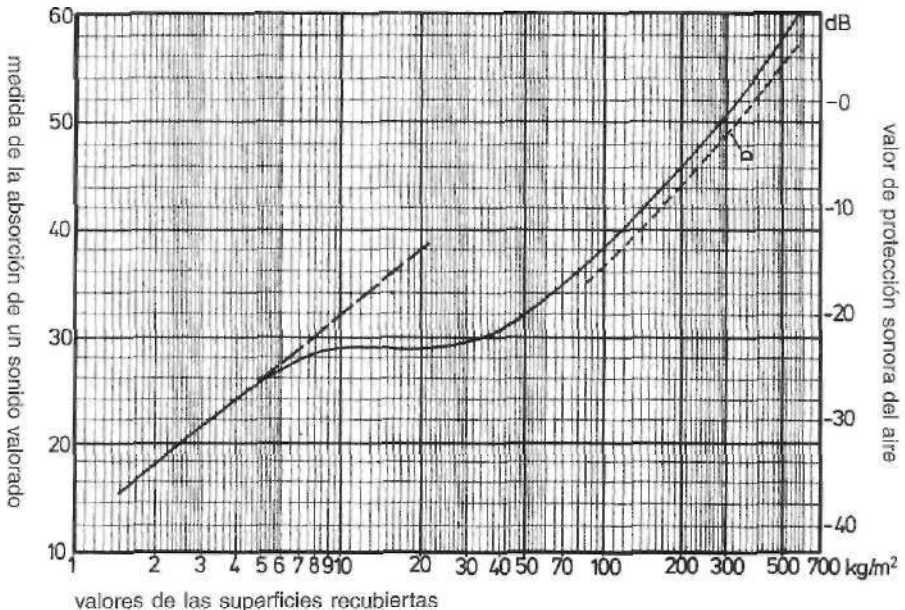
2.6 Dependencia de la aislación acústica del aire con el peso de las superficies (Gosele, Schüle 1983)
