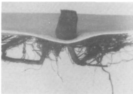
4.6 Perforación en una unión pegada de dos láminas de PVC producida por una raíz (Pennigsfeld et al. 1981)
