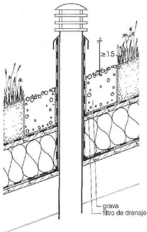
6.16 Encuentro con una ventilación
