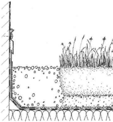
6.3, 6.4 Encuentros de borde con muros que continúan
