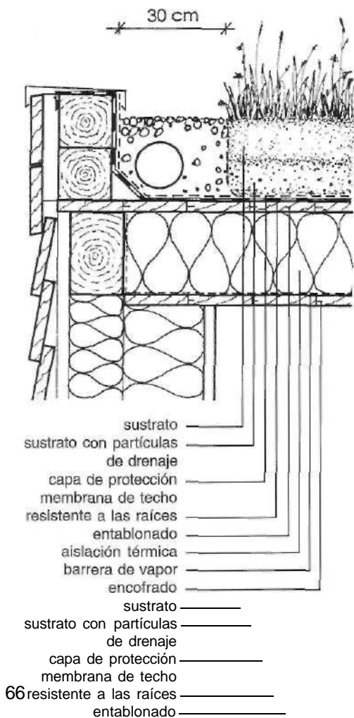
6.6 Construcción del borde de techo con canal
