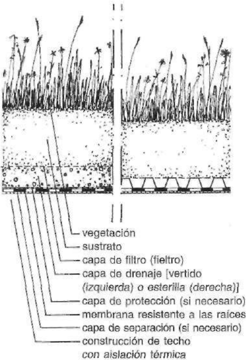
4.1 Construcción de un enjardinado de techo plano con sustrato en dos capas
