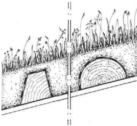
18 Seguridad contra el deslizamiento del sustrato mediante umbrales de empuje
