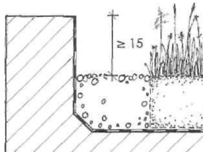
Encuentros de borde con ático ó muro
