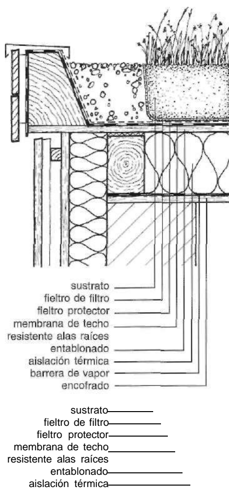
6.7 Construcción del borde de techo con pretil
