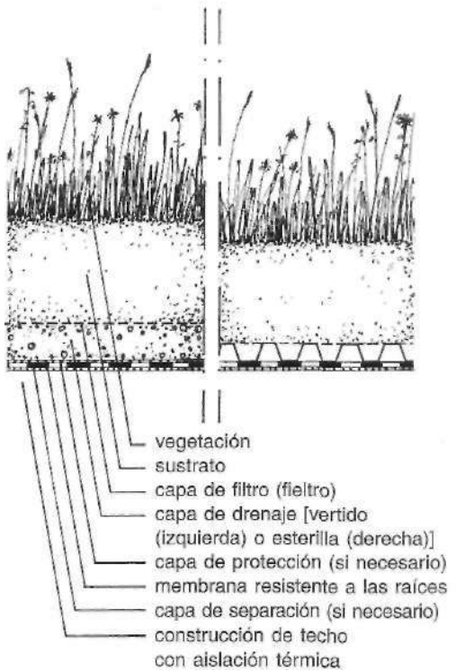
5.2 Construcción en capas de enjardinados para techos planos
