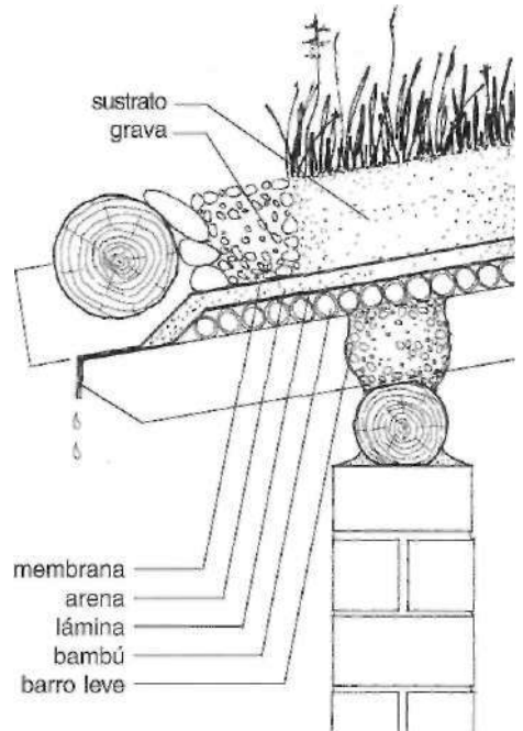
6.12 Detalle de canalón sin drenaje
