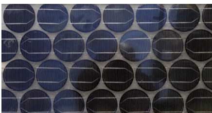
Instalación del Provincial Domain de Chevetogne, desmontada en el 2009, después de 26 años de funcionamiento.
